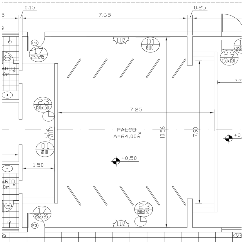
Figura 1 Planta Baixa do Espaço
